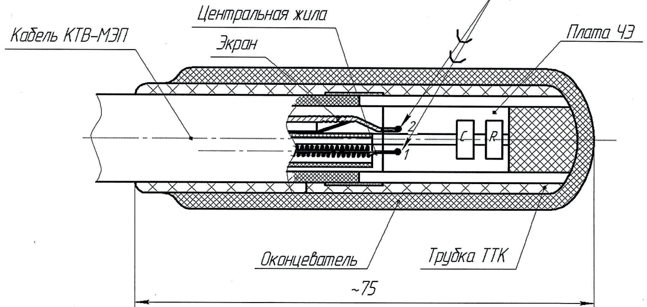
Рисунок 1 – Монтаж ОУ на кабеле СЧЭ КТВ-МЭП
