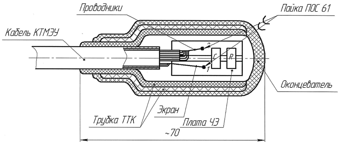
Рисунок 1 – Монтаж ОУ на кабеле ЧЭ
