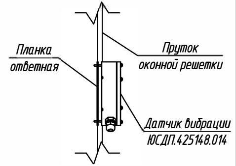
Установка датчика вибрации
