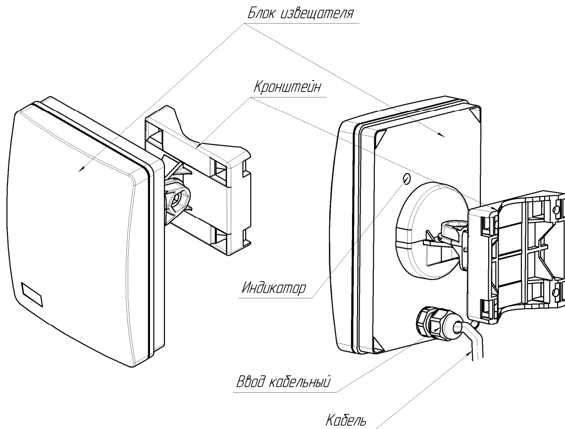
Рисунок 1.2 – Внешний вид блока извещателя
