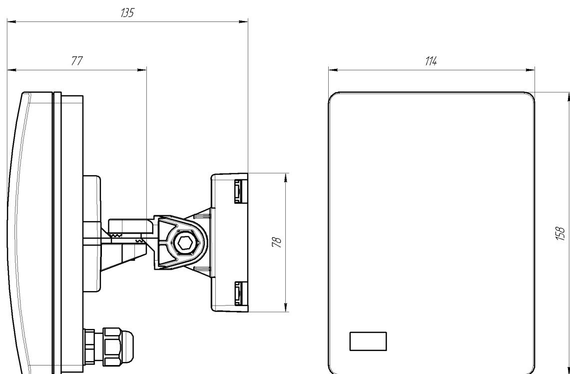
Рисунок 1.3 – Габаритные размеры блока извещателя
