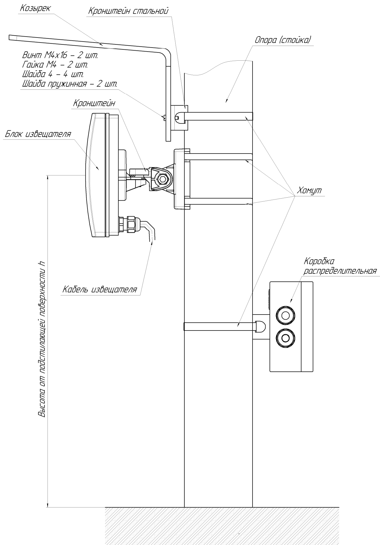
Рисунок 2.1 – Установка извещателя на опоре (высота установки h=1.2\dots1.5 м)
