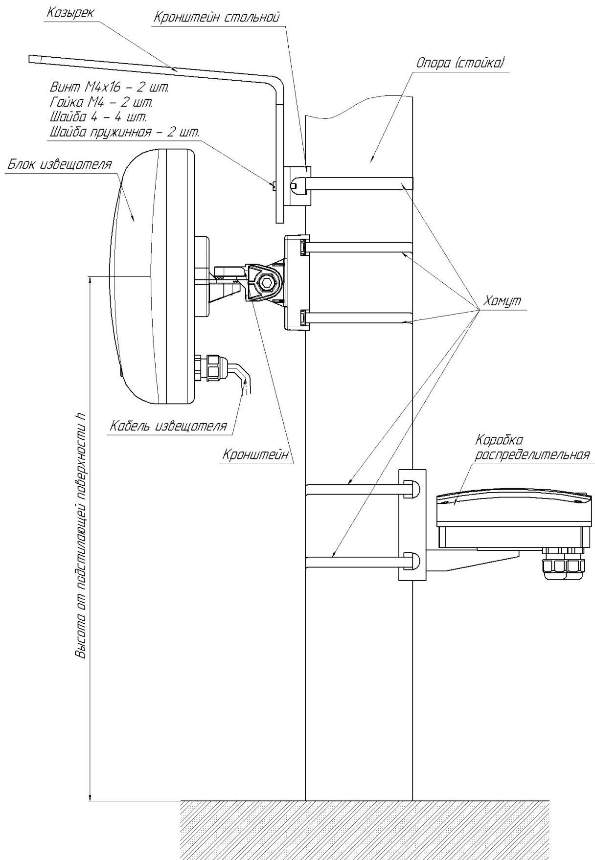
Рисунок 2.1 – Установка извещателя на опоре (высота установки h=1.2...1.5 м)
