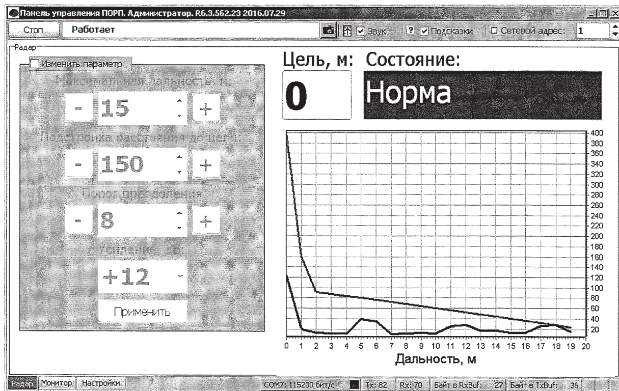
Рисунок А.6 – Вкладка «Радар»
