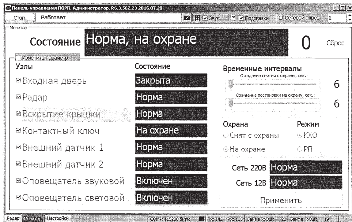
Рисунок А.7 – Вкладка «Монитор»
