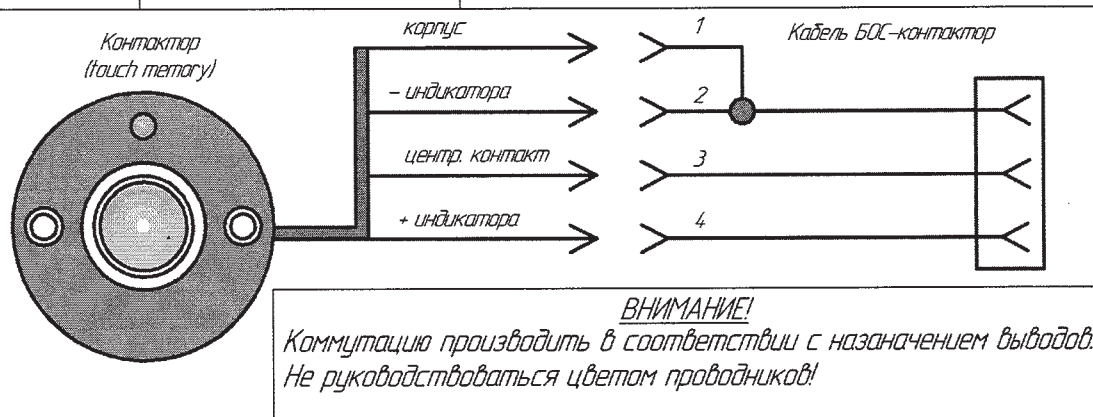
Рисунок 2.4 – Схема подключения контактора
