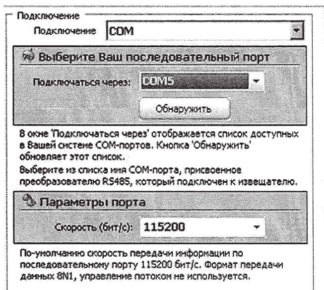
Рисунок 2.7 – Выбор номера порта и скорости передачи
