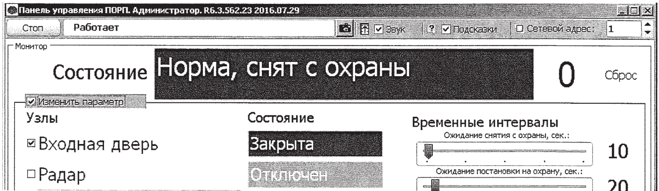
Рисунок 2.12– вкладка «Монитор», РД отключен
