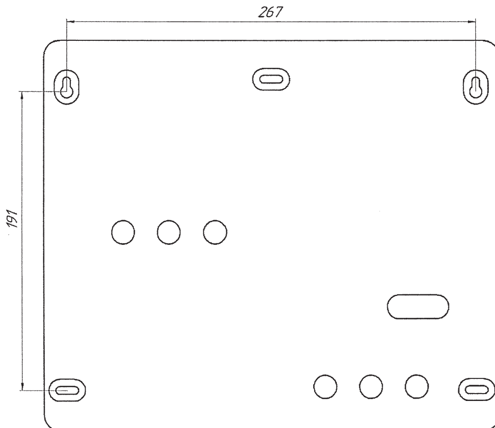
Рисунок 2.1 – Разметка крепления БОС
