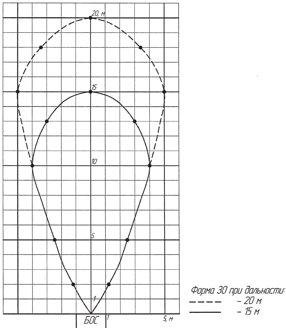
Рисунок 1.3 – Примерный вид ЗО РД БОС, вид сверху
