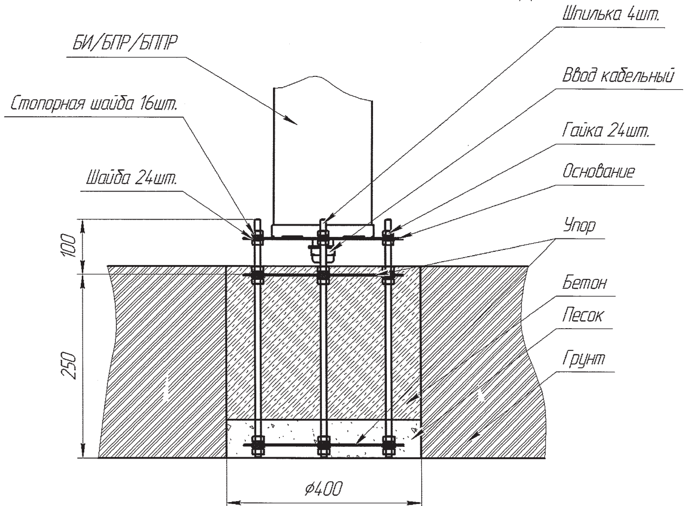
Рисунок 1.5 – Пример установки БИ, БПР, БППР на грунте
