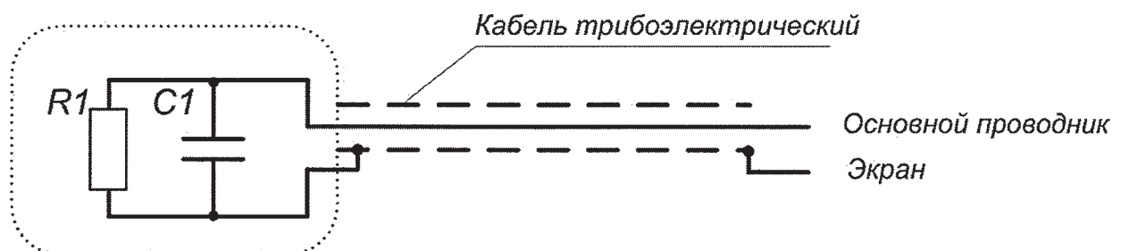
Рисунок 1.6 – Конструкция ВЧЭ
