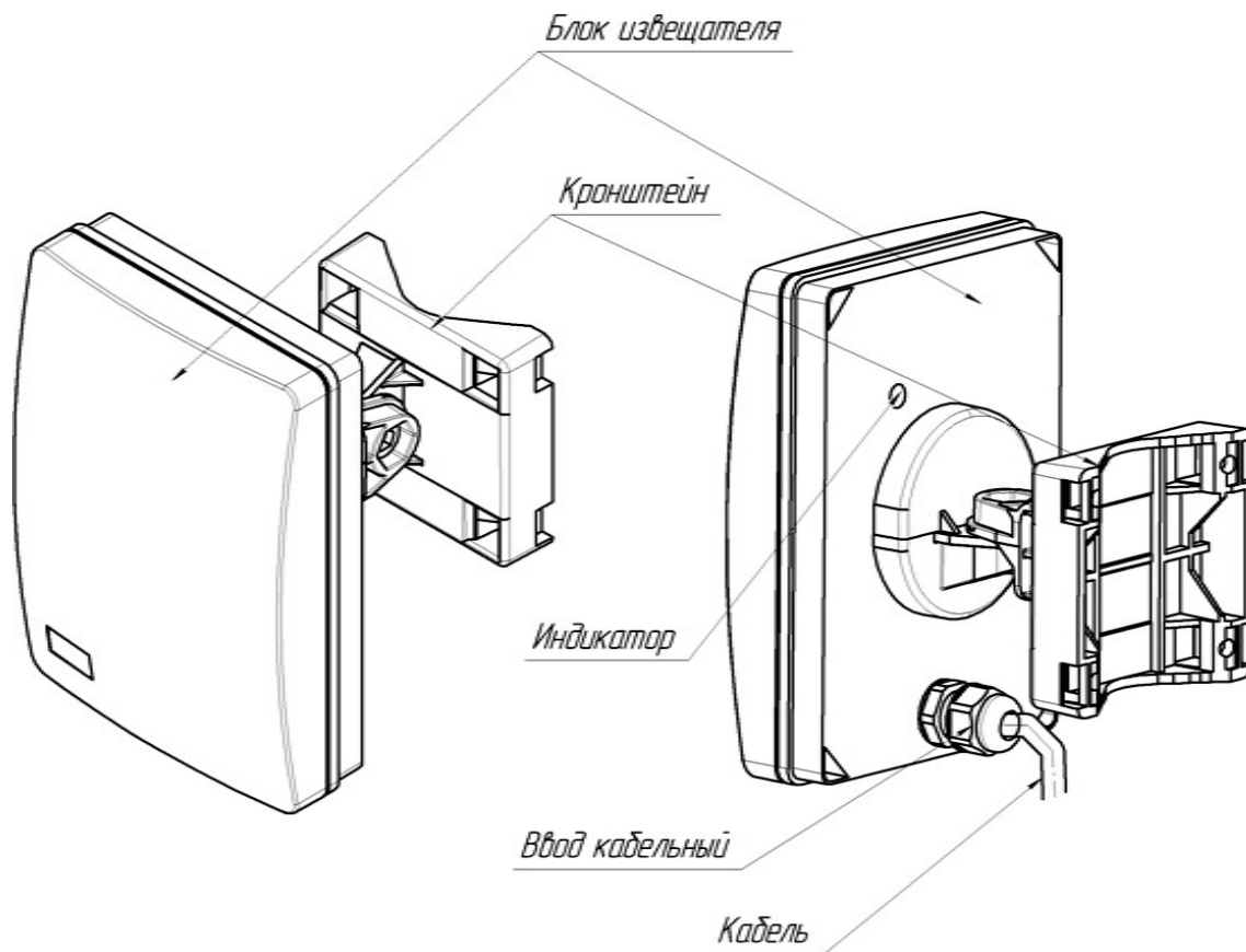
Рисунок 1.3 – Внешний вид блока (ПРМ, ПРД) извещателя
