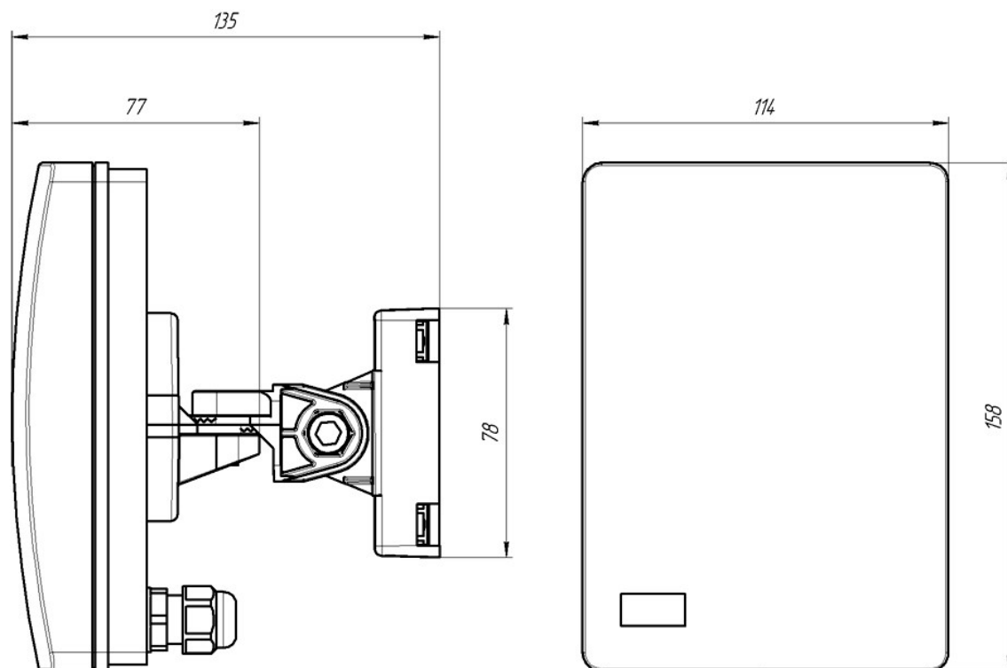
Рисунок 1.4 – Габаритные размеры блока (ПРМ, ПРД) извещателя
