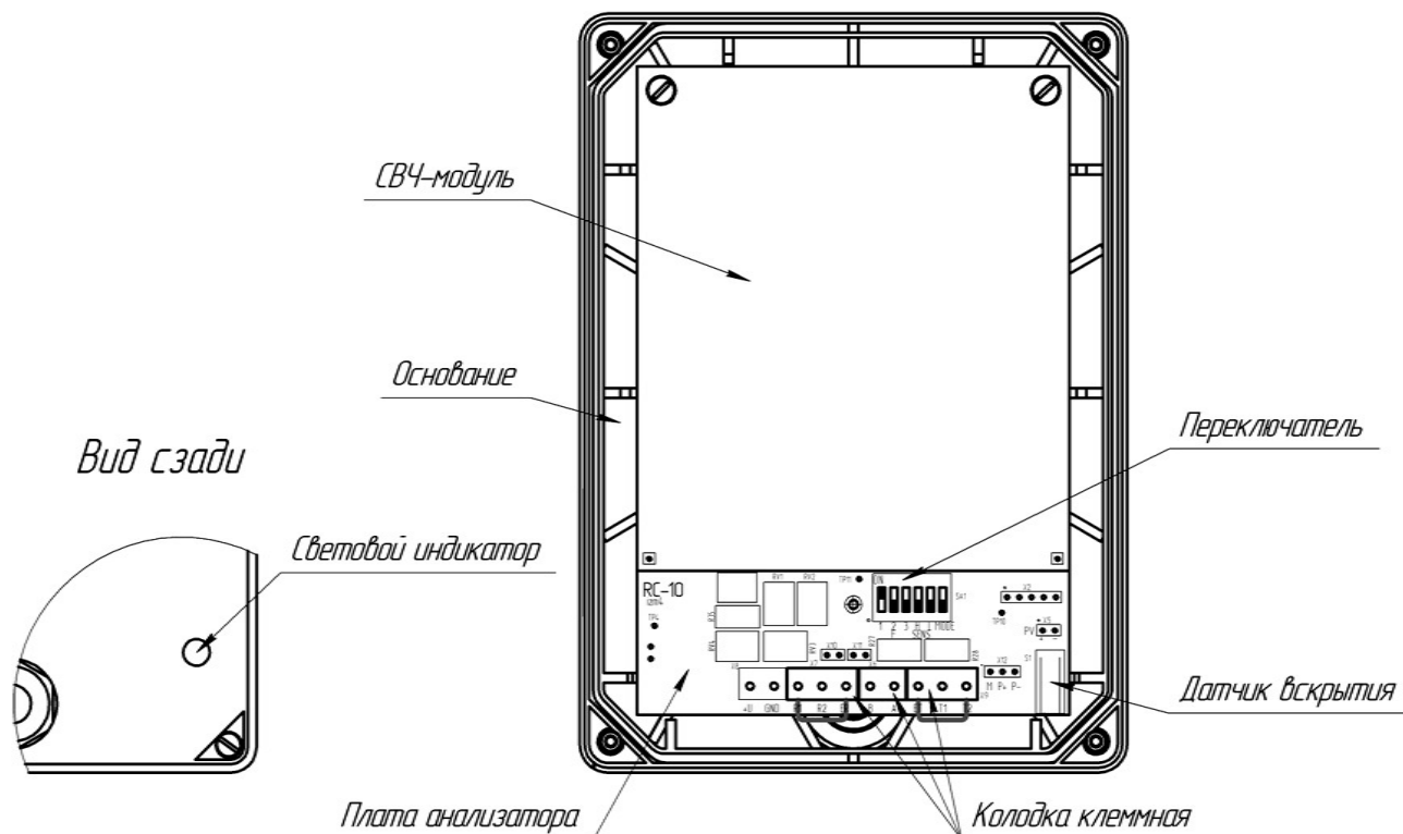
Рисунок 1.6 – Внешний вид блока ПРМ со снятой крышкой
