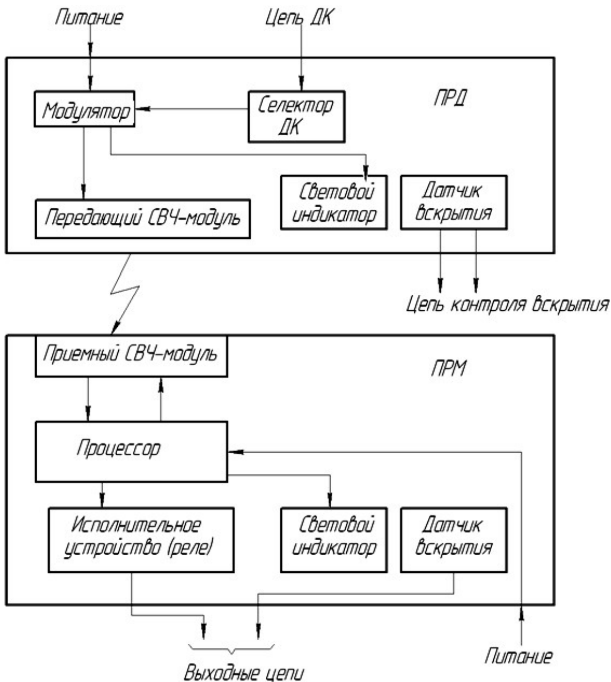
Рисунок 1.2 – Функциональная схема извещателя
