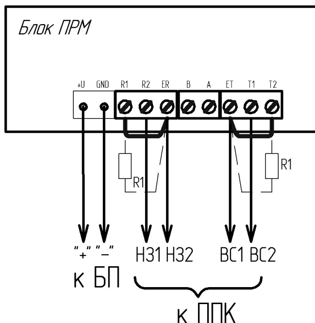
Рисунок 2.6 – Подключение ПРМ с раздельным выводом цепей реле (НЗ) и вскрытия (ВС)
