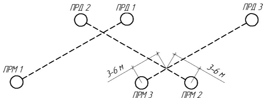
Рисунок 2.3 – Зигзагообразное расположение с перекрытием участков
