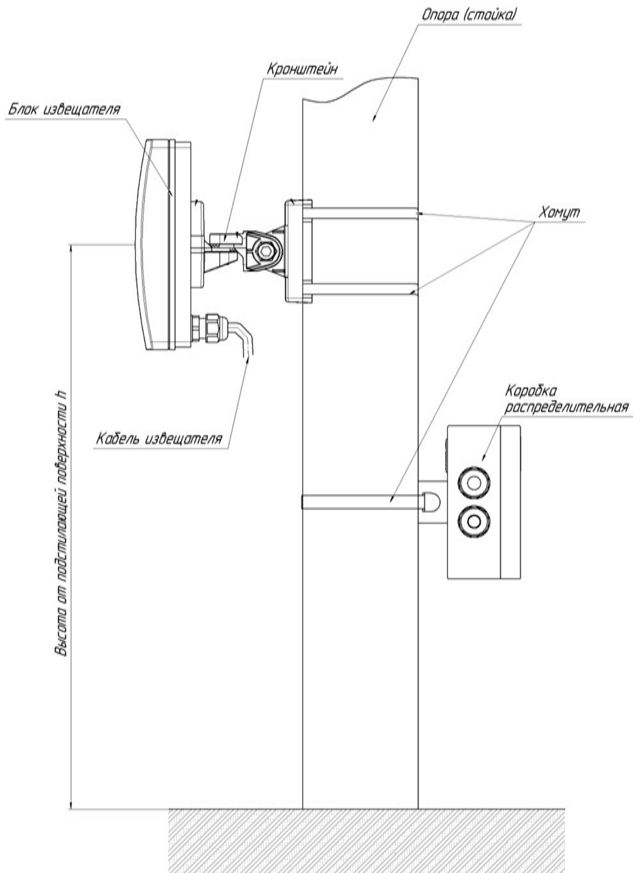
Рисунок 2.5 – Установка блока извещателя и КР на опоре (высота установки h=0.8\ldots0.9 м)
