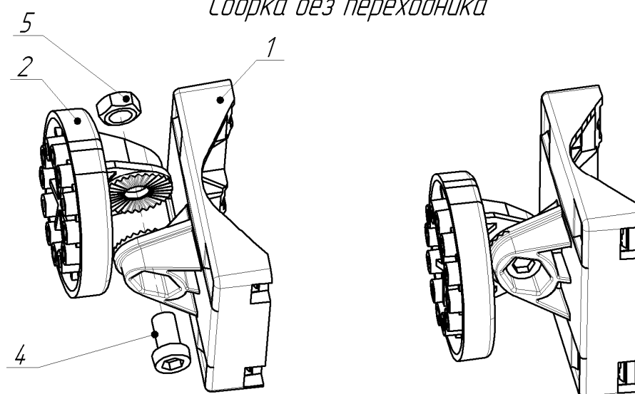
Сборка без переходника
