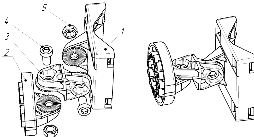
Сборка без переходника
