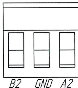
Рисунок 2.6 – Внешний вид колодки клеммной «Порт 2» ПИ
