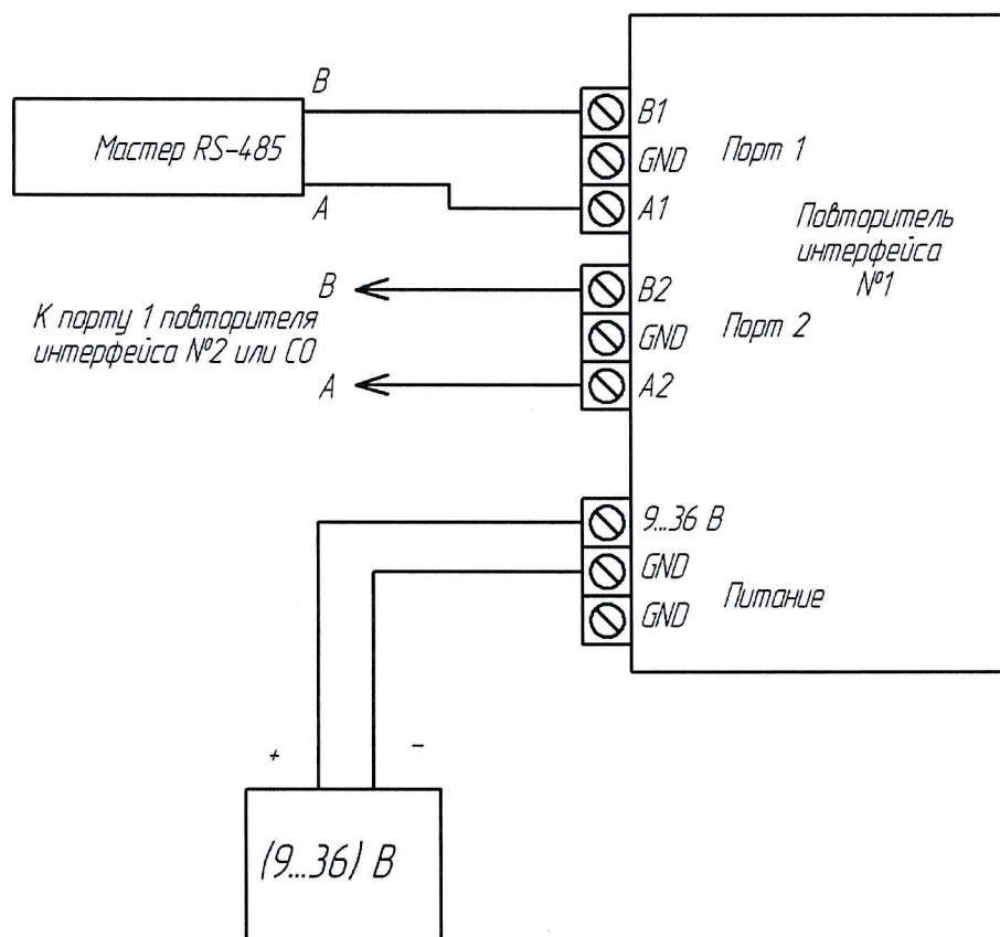
Рисунок 2.3 – Схема подключения ПИ
