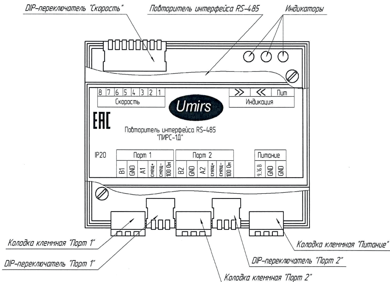
Рисунок 2.1 - Внешний вид ПИ RS-485
