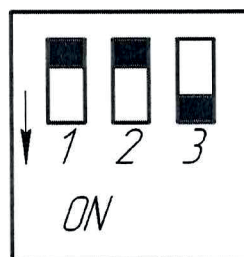
Рисунок 2.8 – Положение переключателей при активации смещающих и терминирующего резисторов
