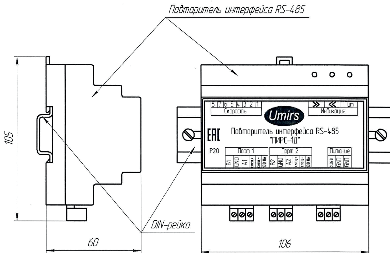
Рисунок 2.2 – Установка ПИ на DIN-рейку
