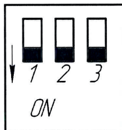
Рисунок 2.9 – Положение переключателей при активации смещающих и терминирующего резисторов
