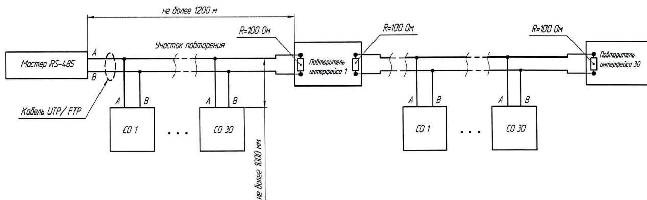
Рисунок 2.10 – Пример организации линии интерфейса
