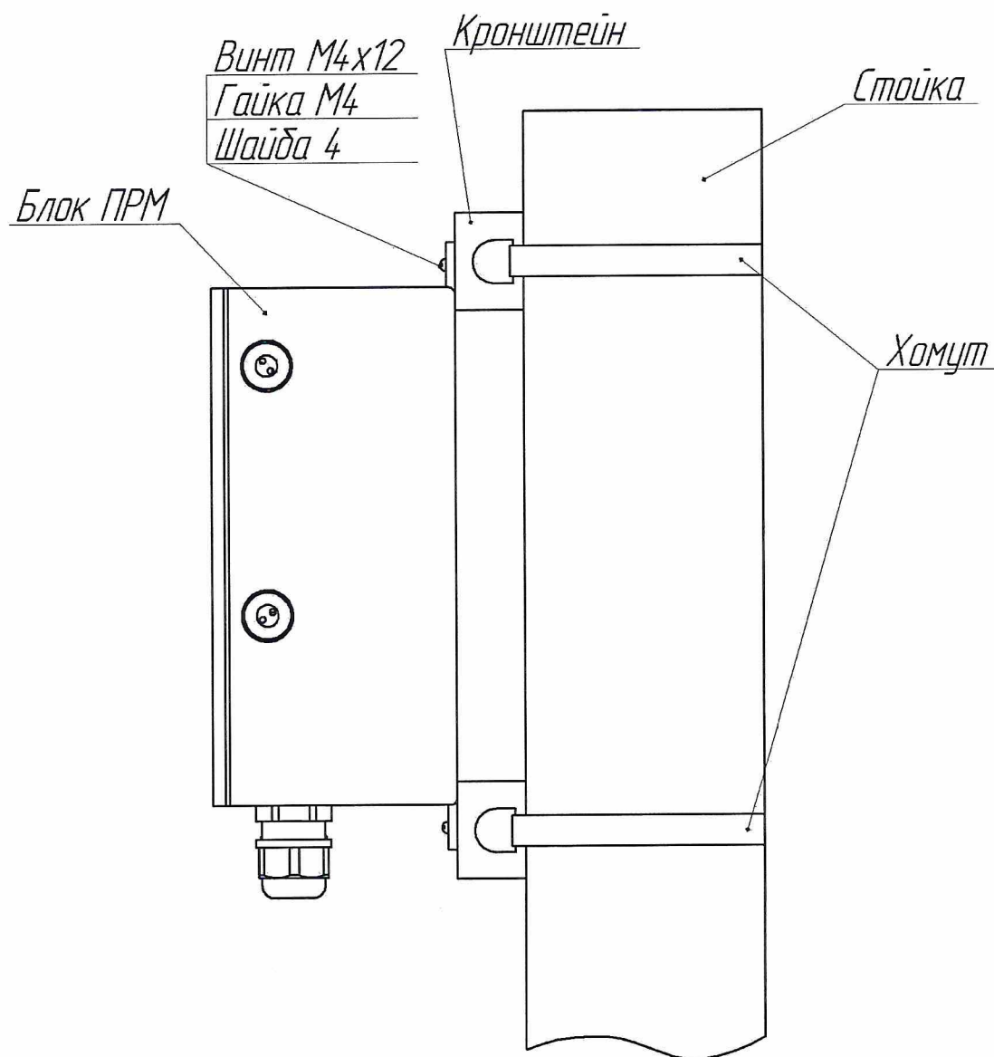
Рисунок 2.1 – Установка блока ПРМ/ПРД на опоре (стойке)
