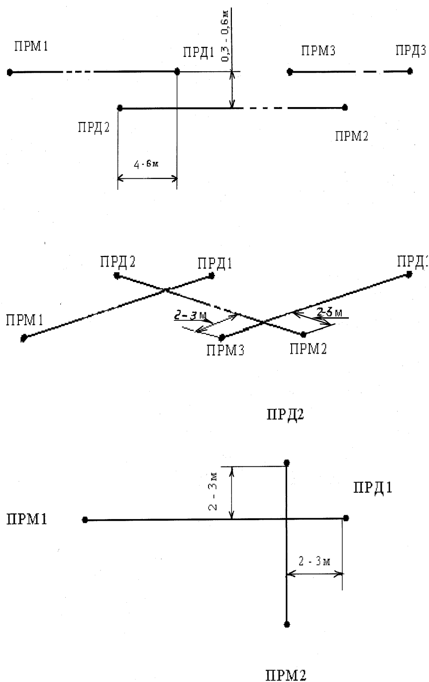
Рисунок В.1 – Примеры установки извещателей
