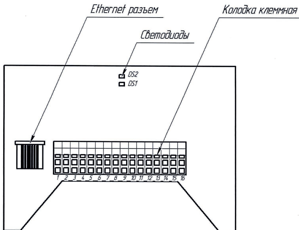
Рисунок 2.5 – Внешний вид платы управления реле
