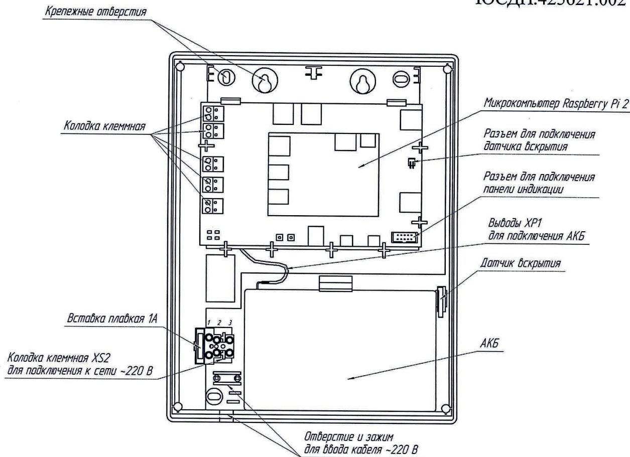
Рисунок 1.2 – Внешний вид БСУ с открытой крышкой (крышка не показана)
