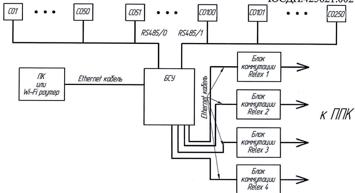
Рисунок 1.4 – Структурная схема подключения изделия к ППК по выходу реле
