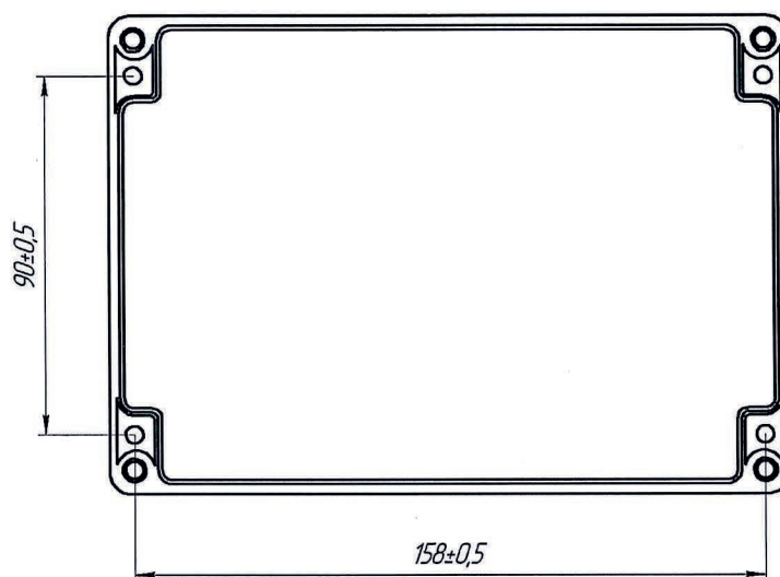
Рисунок 2.2 – Разметка крепления блока коммутации
