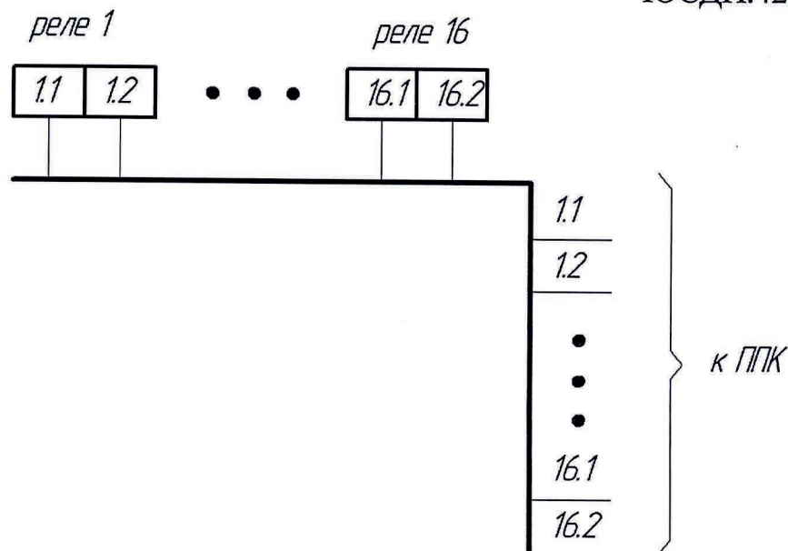
Рисунок 2.6 – Коммутация блока коммутации с ППК
