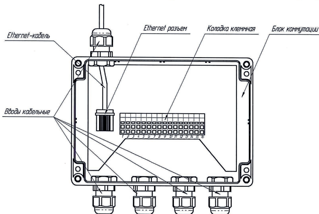
Рисунок 1.3 – Внешний вид блока коммутации (крышка не показана)
