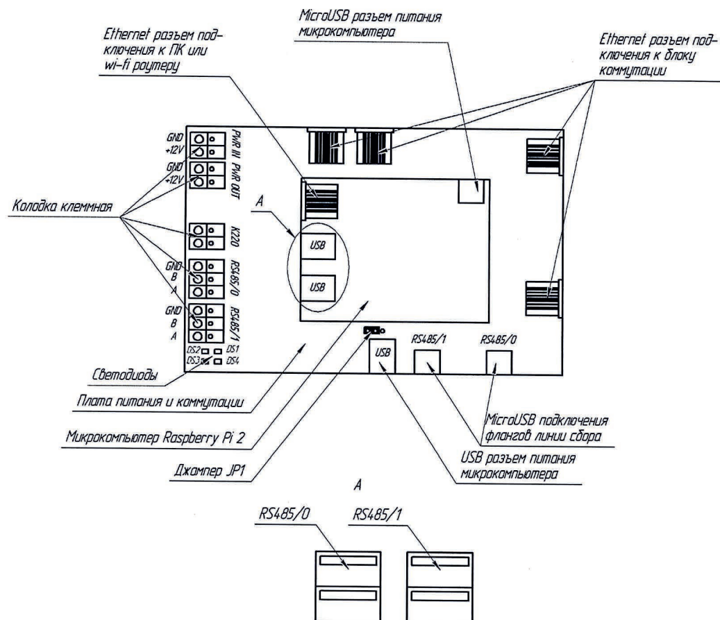
Рисунок 2.3 – Внешний вид платы питания и коммутации с микрокомпьютером
