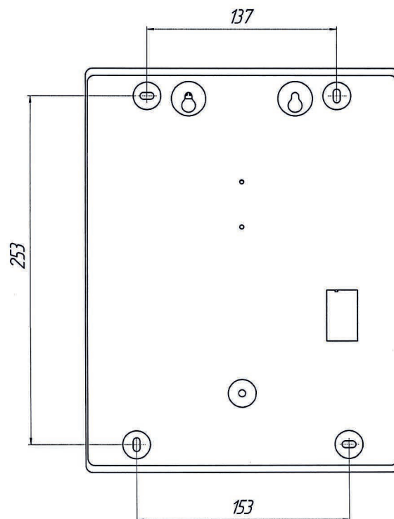
Рисунок 2.1 – Разметка крепления БСУ
