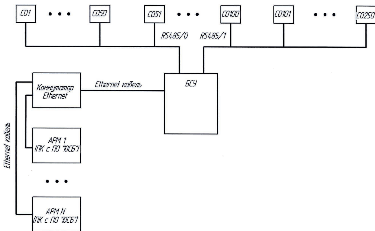
Рисунок 1.5 – Структурная схема подключения изделия к ПК с ПО «ЮСБ»
